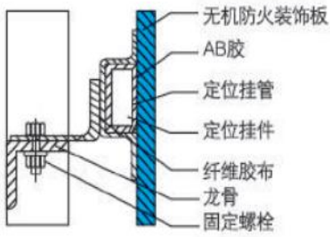
DPX无机防火装饰板安装示意图
